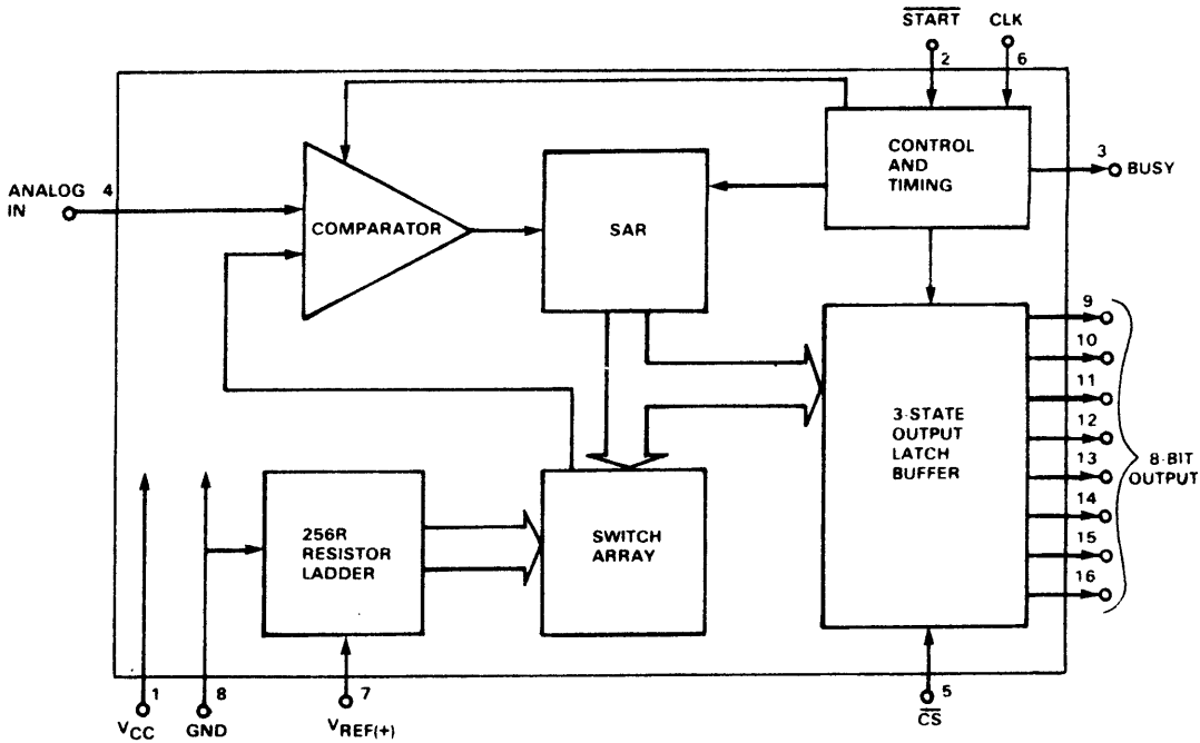
2.ábra: MK 5168 blokkvázlata
