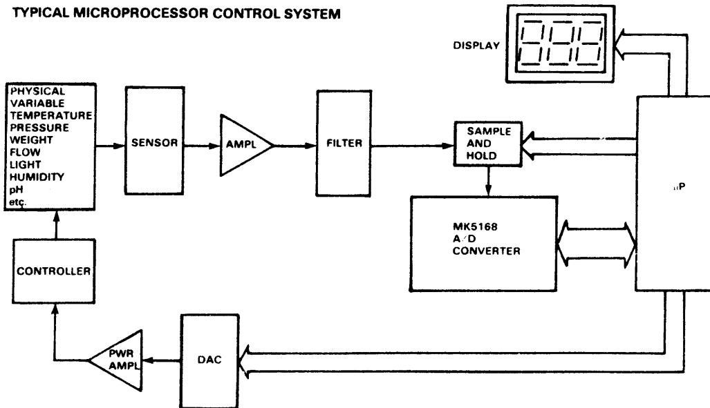
3.ábra: Tipikus CPU vezérelt rendszer felépítése
